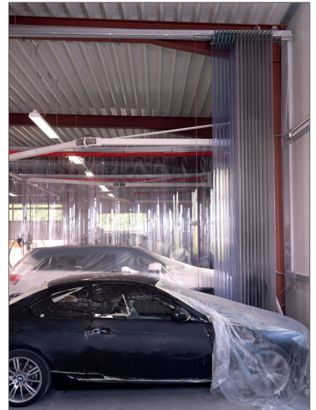
Arbeitsplätze 4 und 5: QUICK-STRIP Scherenfaltsystem geöffnet Wenn keine Nischen zum Verschieben des Streifenvorhangs vorhanden sind, werden die einzelnen Streifen um 90° gedreht und auf kleinstem Raum gestapelt.
