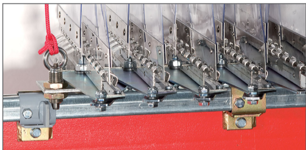
QUICK-STRIP Scherenfaltsystem
